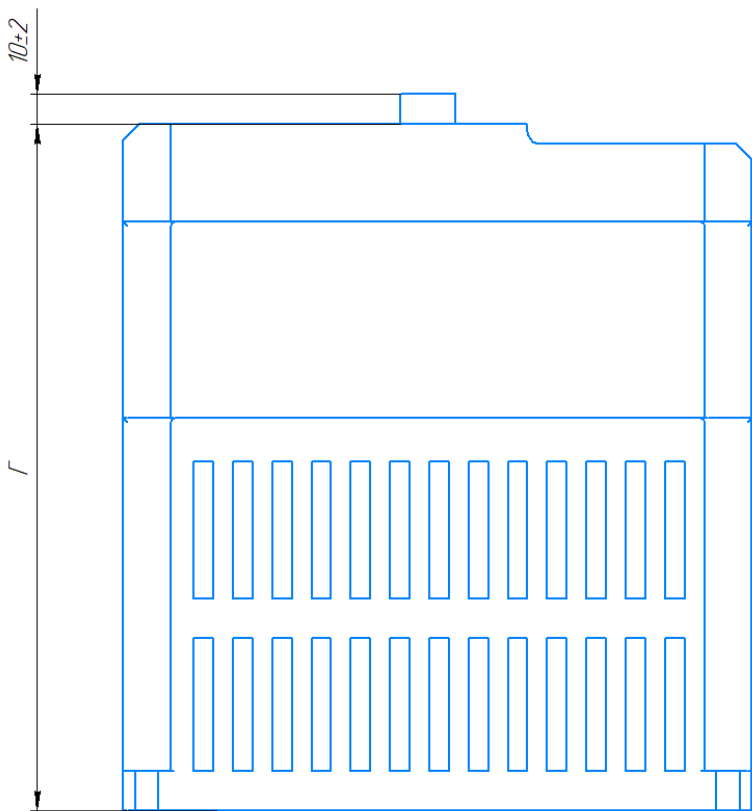
Рис. 2.5.26 - габаритные и установочные размеры устройств серии LCI в пластмассовом корпусе
