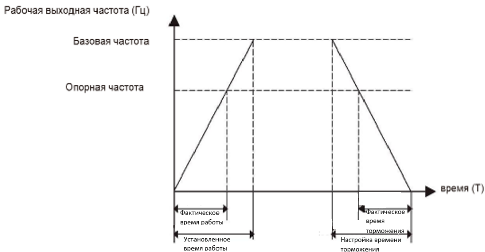
Рисунок 6-1 Время разгона/торможения
