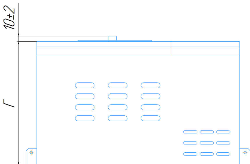
Рис. 2.5.3а – габаритные и установочные размеры LCI в металлическом корпусе
