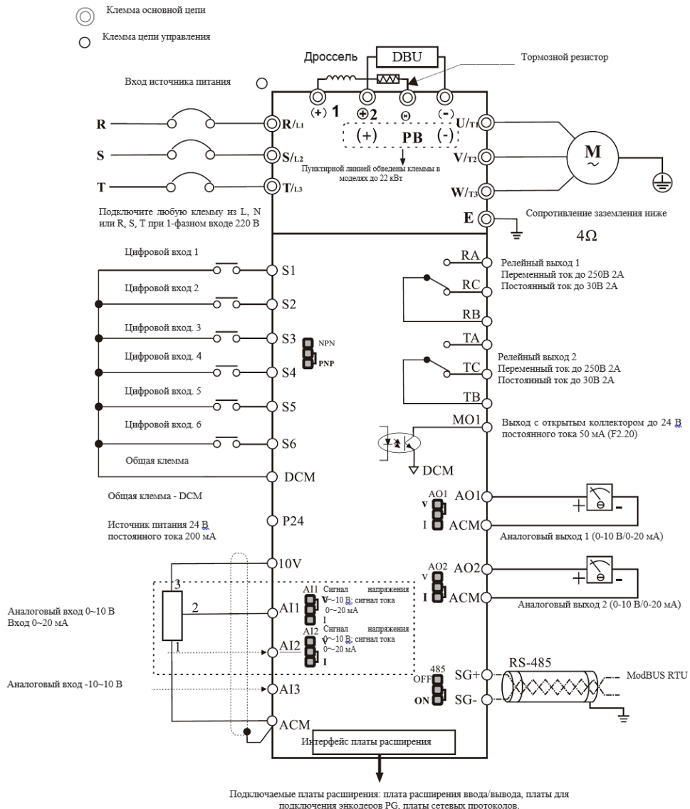
Рис. 4.5.1 – Схема подключения к плате управления LCI
