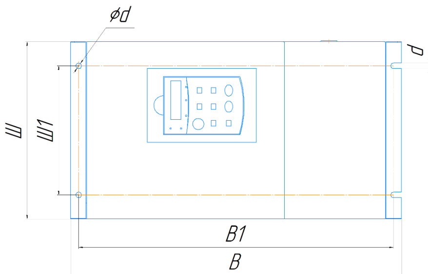
Рис. 2.5.3б – габаритные и установочные размеры LCI в металлическом корпусе
