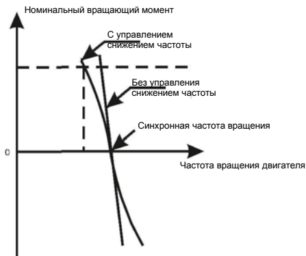
Рис. 6-21. Управление снижением частоты
