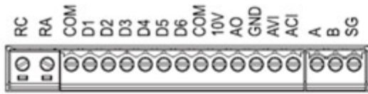
Типоразмер А (А1/А2) SP5L...S3L, 001H...003H
