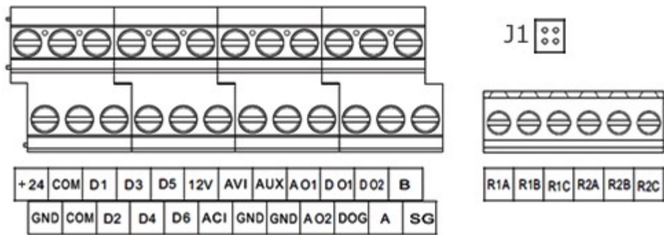
Типоразмер Е, F, G, H, I, J 040H...400H
