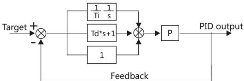
Рисунок 6-34 Принципиальная блок-схема ПИД-регулирования
