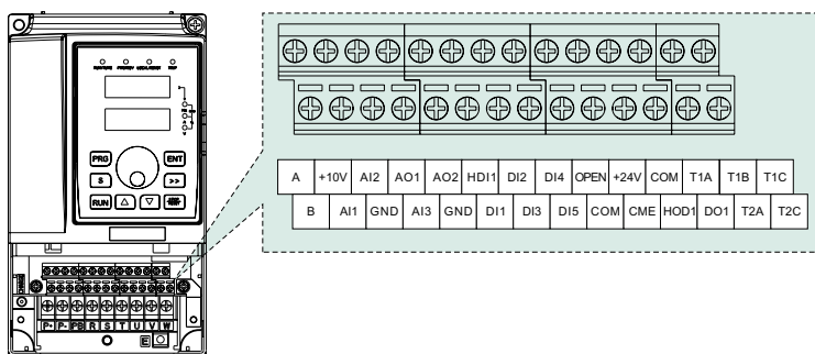
Рисунок 3-17. Клеммы управления.
