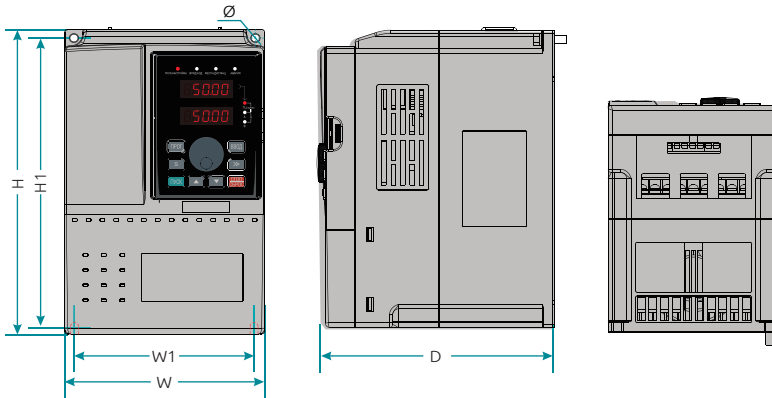
Рисунок 2-б. Установочные размеры ПЧ мощностью до 7,5 кВт (включительно)
