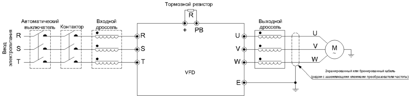
Рис. 3-3.1. Схема подключения преобразователя частоты
